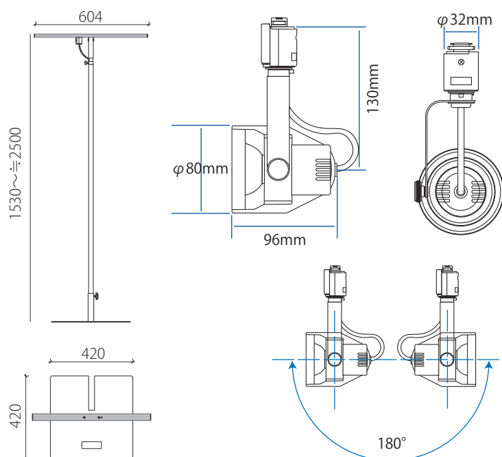
Profile sketch 製品姿図
