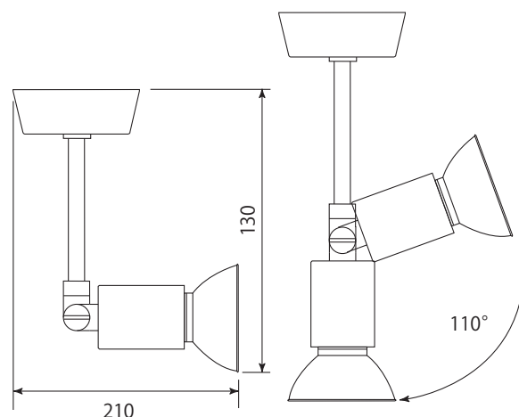
Profile sketch 製品 姿図
