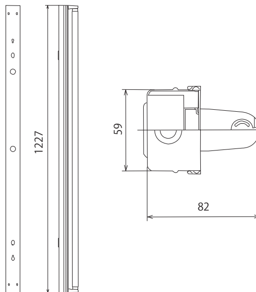
Profile sketch 製品姿図
