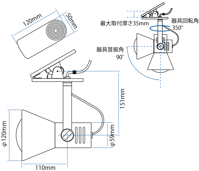
Profile sketch 製品 姿図
