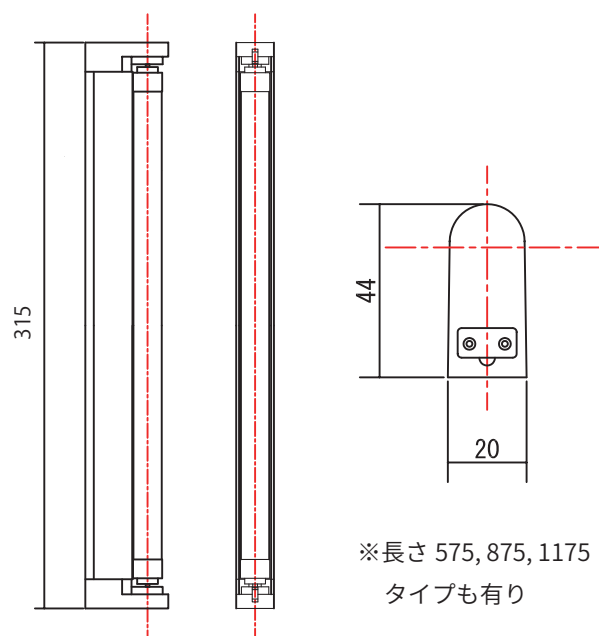
Profile sketch 製品姿図
