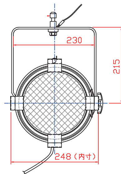
Profile sketch 製品姿図
