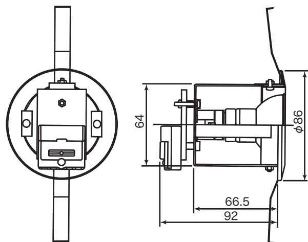
Profile sketch 製品姿図
