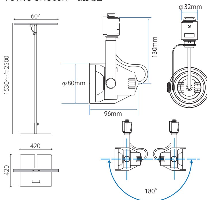
Profile sketch 製品 姿図
