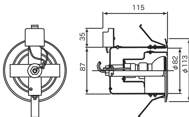
Profile sketch 製品姿図
