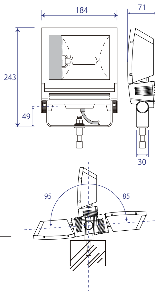
Profile sketch 製品 姿図
