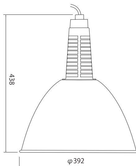
Profile sketch 製品姿図
