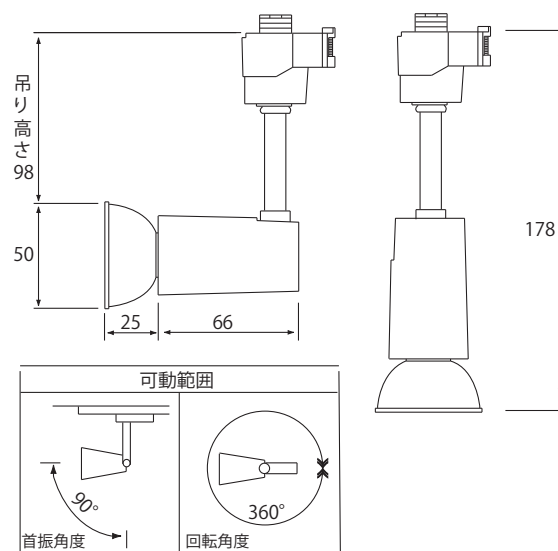
Profile sketch 製品 姿図
