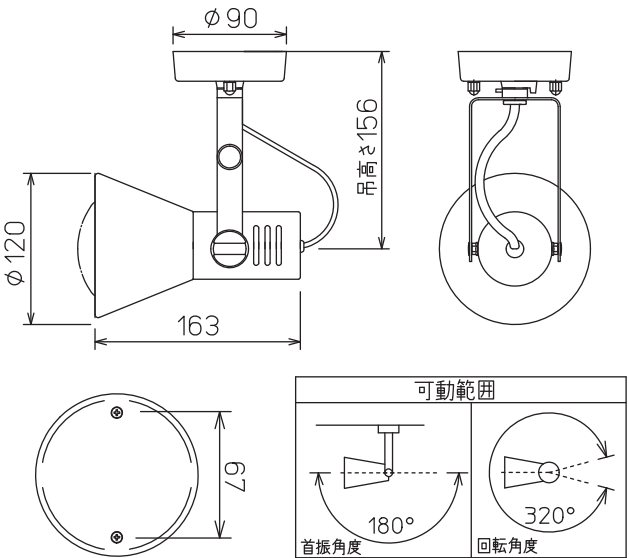
Profile sketch 製品 姿図
