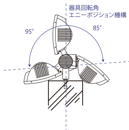
Fitting 取付方法
