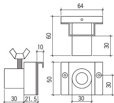
オクタ金具 (ネジ付き)
