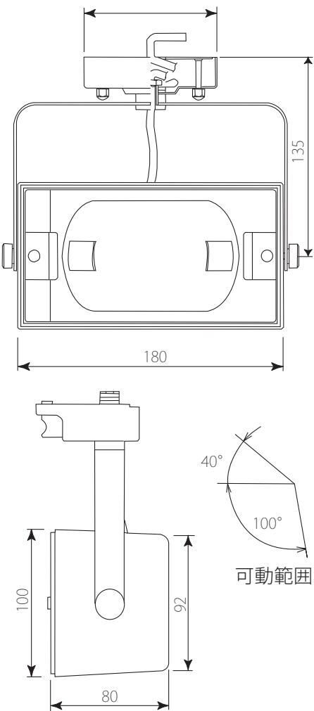
Profile sketch 製品 姿図
