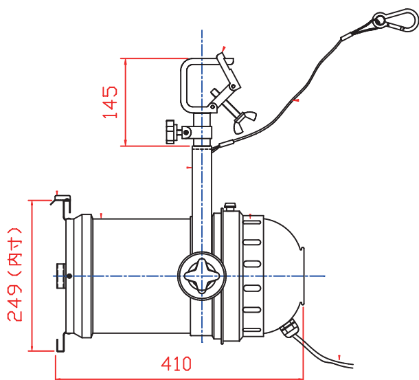
Fitting 取付方法 Fitting profile sketch 取付方法 姿図
