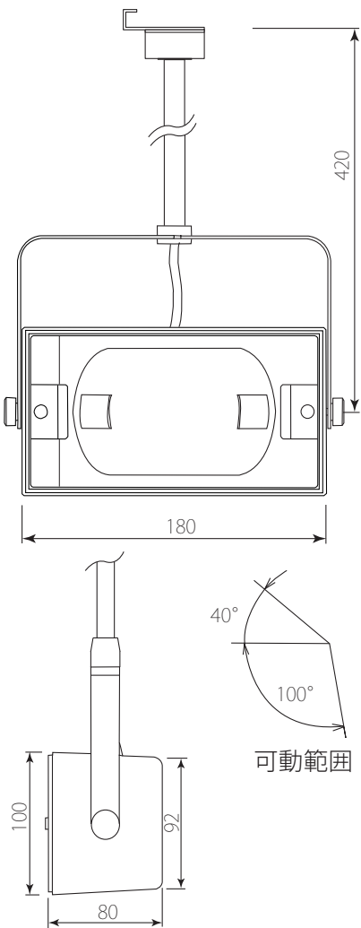
Profile sketch 製品 姿図
