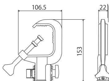
Fitting 取付方法 Fitting profile sketch 取付方法 姿図
