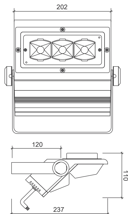
Profile sketch 製品 姿図
