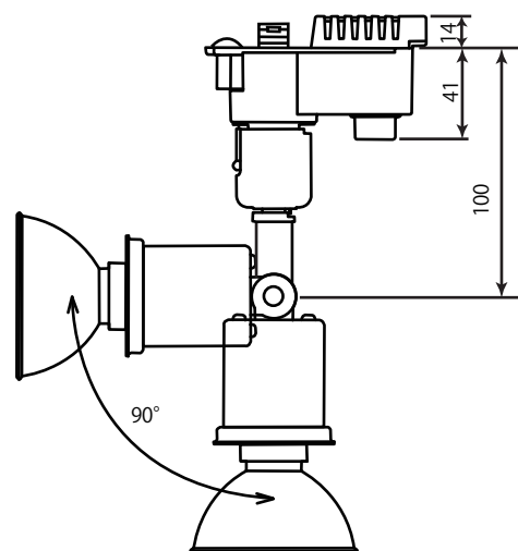
Profile sketch 製品 姿図
