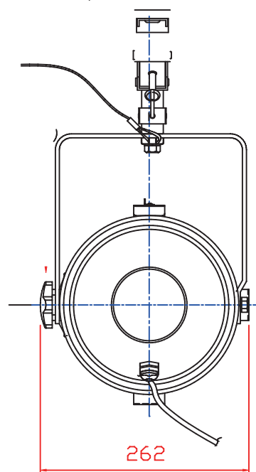
Fitting 取付方法 Fitting profile sketch 取付方法 姿図
